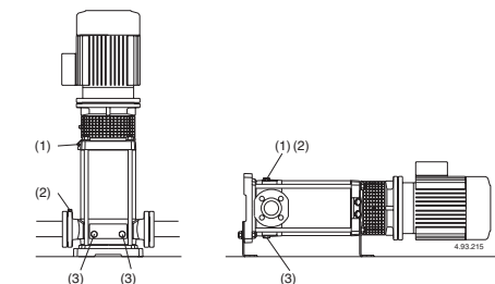
Fig. 4d (1) Fyllning samt luftskruv
