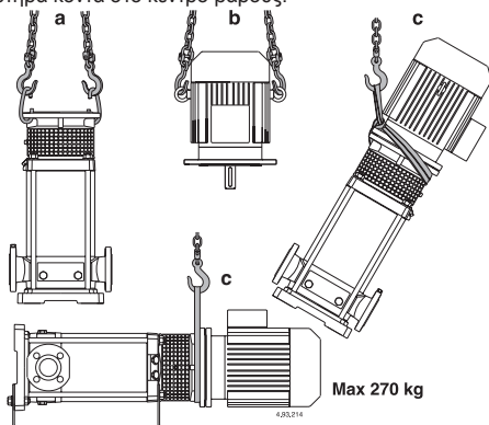
Σχ.1 α Ανύψωση της ανλίας χωρίς μοτέρ β Ανύψωση της κινητήρα χωρίς αντλία c Ανύψωση της ανλίας με μοτέρ
