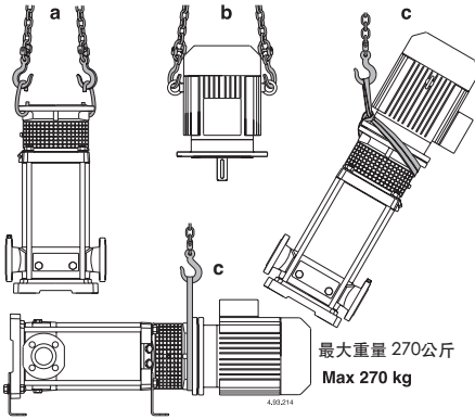
图 1 a 泵的提升 b 电机的提升 c 泵组的提升
