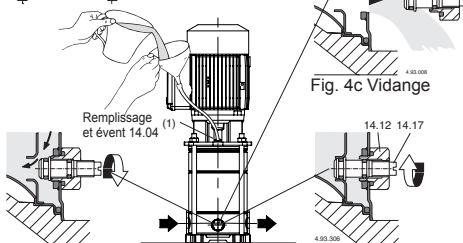
Fig. 4a Remplissage: passage intérieur ouvert
