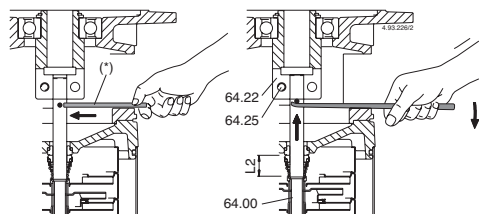
Σχ.6α Σταθεροποίηση ρότορα με απα- σφαλισμένο άξονα στην σύζευξη. (*) Σφήνα για ανύψωση του άξονα.
