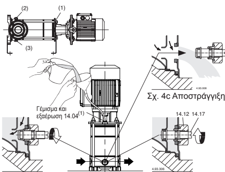
Σχ. 4α Γέμισμα: εσωτερική διόδος ανοίγματος Σχ. 4β Χειρισμός: εσωτερική διόδος κλεισίματος
